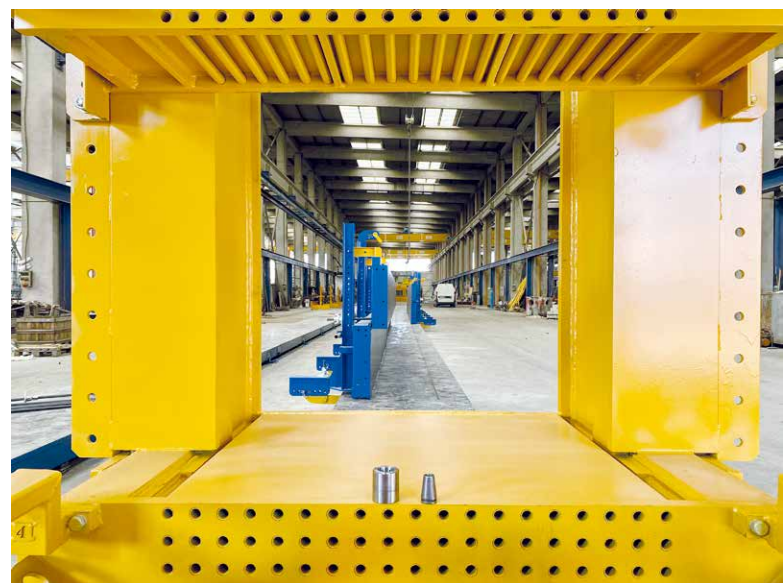
68 米长的应力头底座，和生产 T 形、L 形和矩形梁的侧面模具
